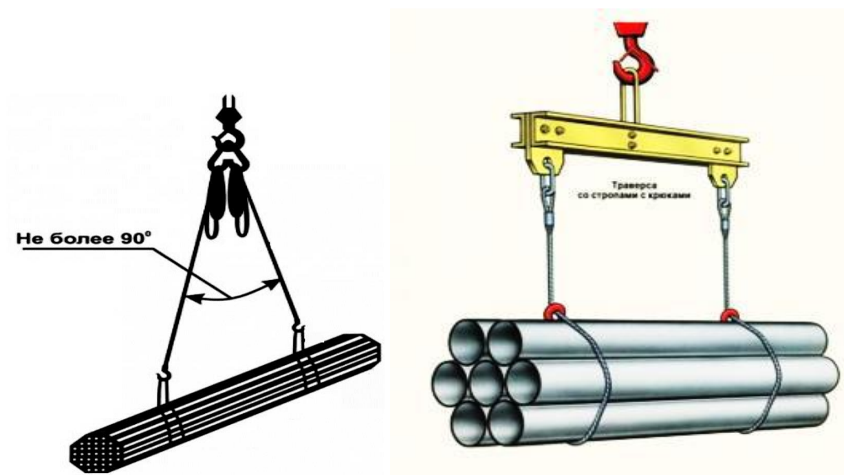
Рис.3.1 – Схемы строповки труб
