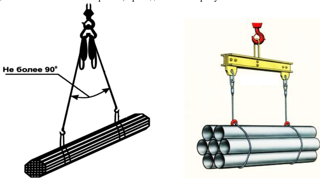
Рисунок 3.1 – Схемы застропки труб
